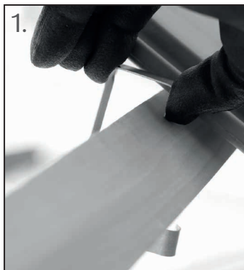
1. Klammer von oben auf die Traglattung stecken ... Place the clip onto the batten ...
